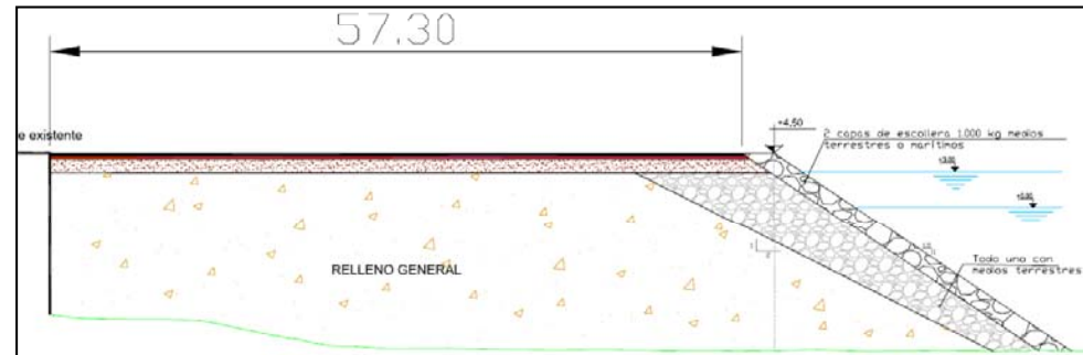
Sección Talud
